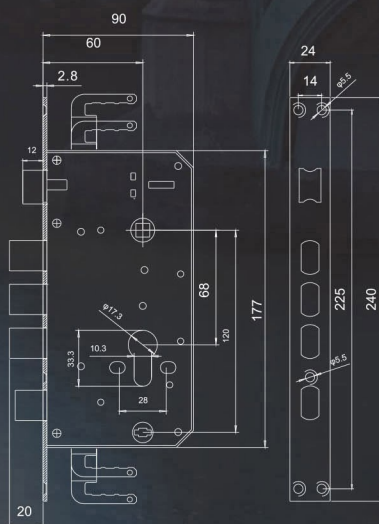
29#全钢多功能锁体安装尺寸
